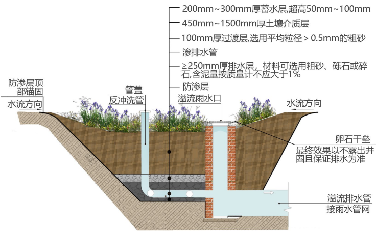
图 5.2-33 雨水花园典型构造示意图
